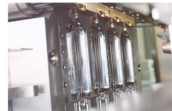
大容量容器产品模具 LVP Mould
